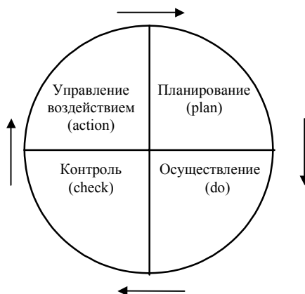
Рис. 3.5. Цикл Деминга
