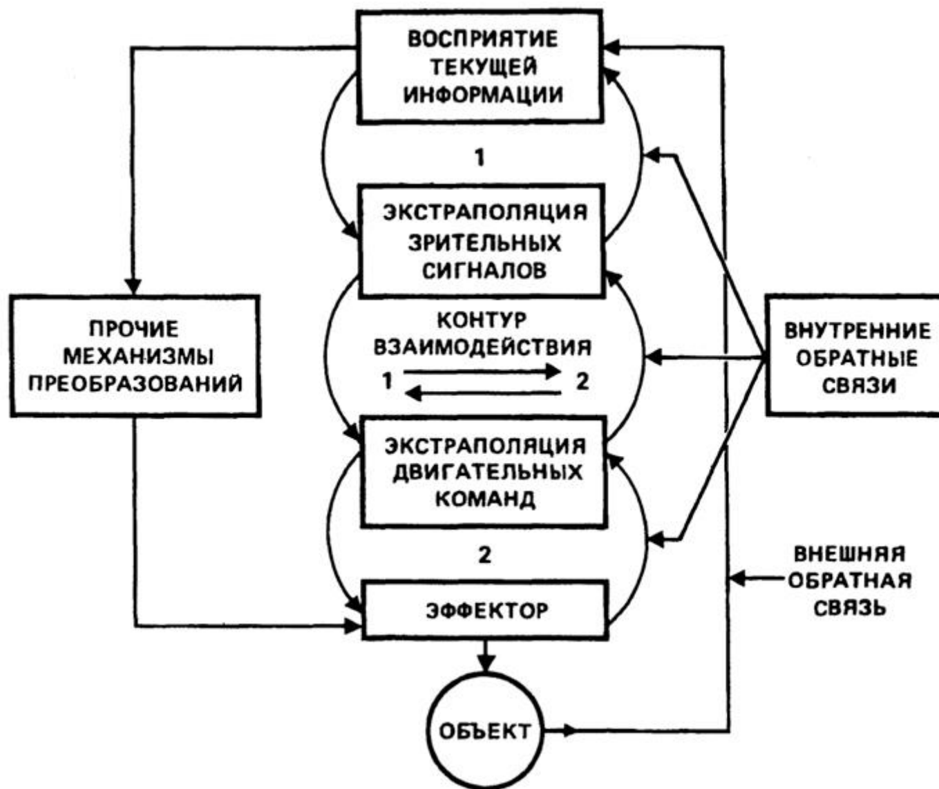
Рис. V.4. Схема взаимодействия замкнутых контуров регулирования, участвующих в управлении движением
